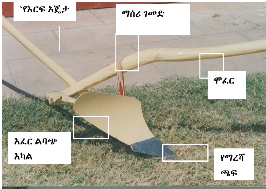
ከእርፍና ሞፍር ጋር የሚገጠም ገልባጭ ማረሻ የሚያሳይ ምስል
