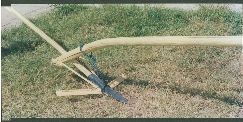
ባለ ክንፍ ማረሻ የሚያሳይ ምስል
